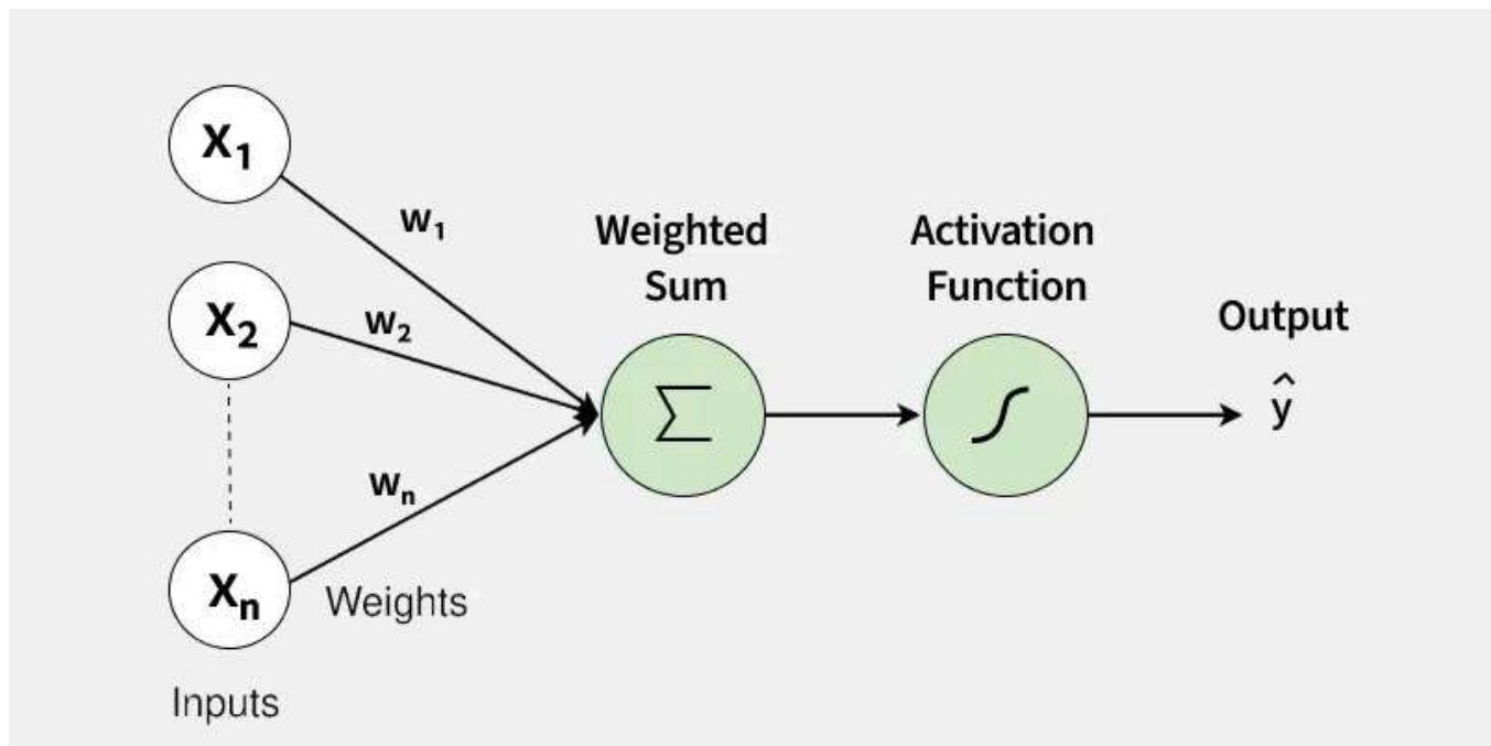
Perceptron
